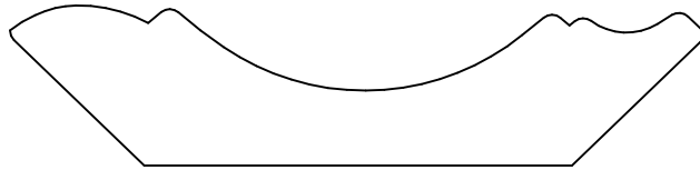
KL 307 .750 x 3.250 2.313 2.313
